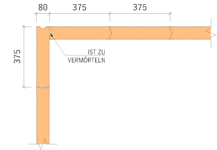
- ECKVERBUND, 2. REIHE DES MAUERWERKS
