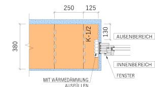
- VERBUND AN DER FENSTERLAIBUNG, 2. REIHE DES MAUERWERKS
