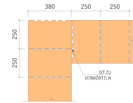
- ECKVERBUND, 1. REIHE DES MAUERWERKS
