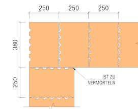
- ECKVERBUND, 2. REIHE DES MAUERWERKS
