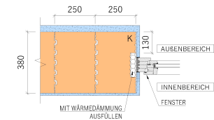
- VERBUND AN DER FENSTERLAIBUNG, 1. REIHE DES MAUERWERKS
