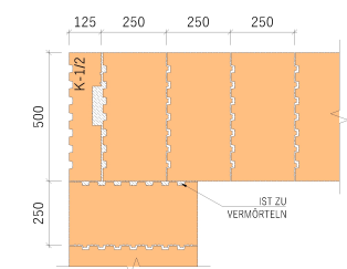
- ECKVERBUND, 2. REIHE DES MAUERWERKS
