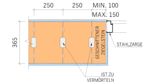
- VERBUND AN DER TÜRLAIBUNG, 2. REIHE DES MAUERWERKS
