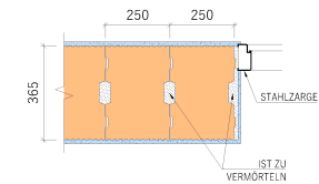
- VERBUND AN DER TÜRLAIBUNG, 1. REIHE DES MAUERWERKS
