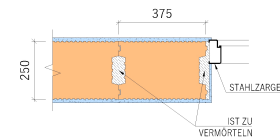
- VERBUND AN DER TÜRLAIBUNG, 1. REIHE DES MAUERWERKS
